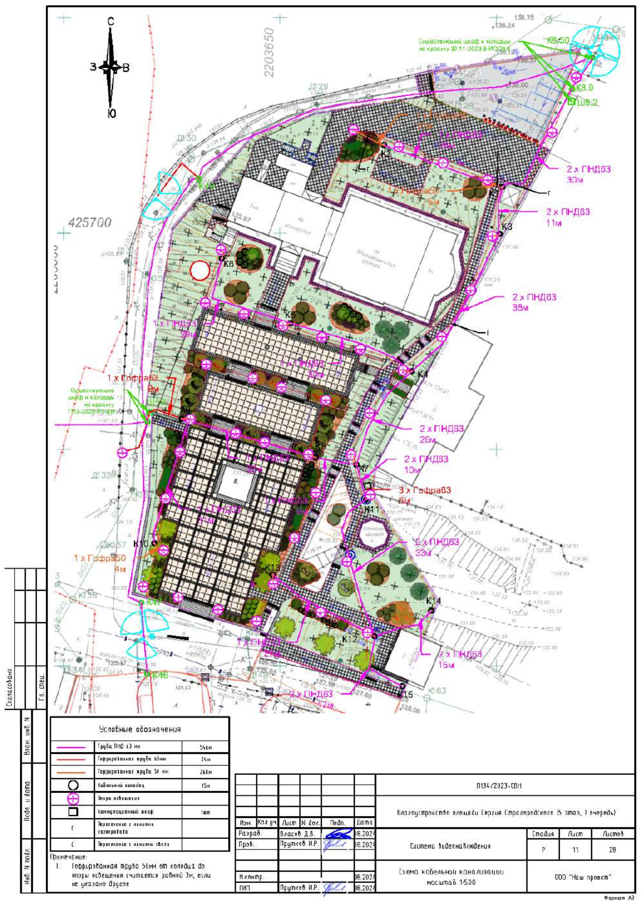
Рис.12. Схема кабельной канализации масштаб 1:500 П134/2023СВН
