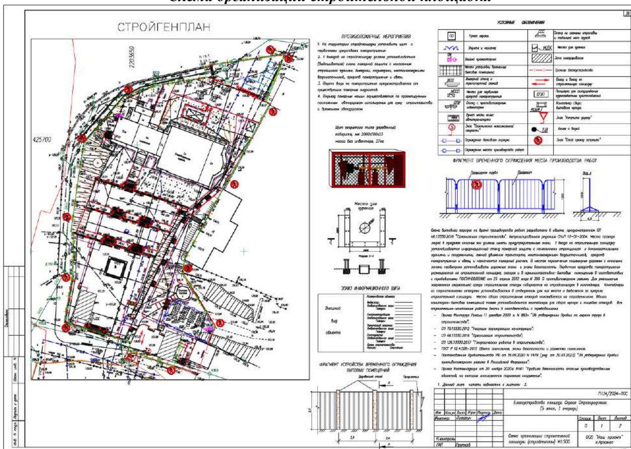
Рис.8. Схема организации строительной площадки (стройгенплан) М1:500. П134/2024-ПОС
